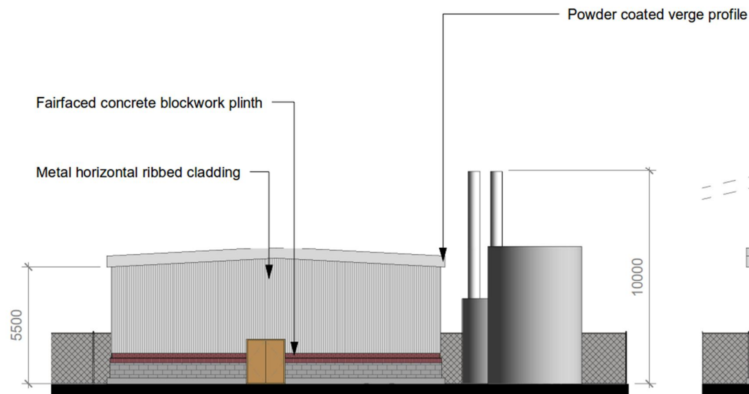
SE Elevation 1 : 200
