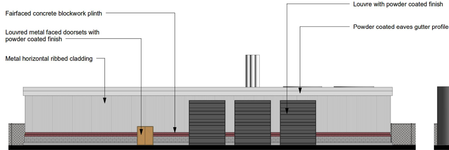
SW Elevation 1 : 200
