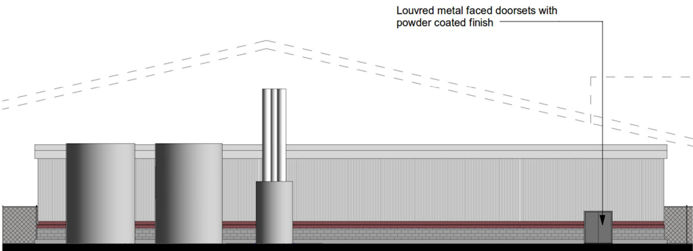
NE Elevation 1 : 200
